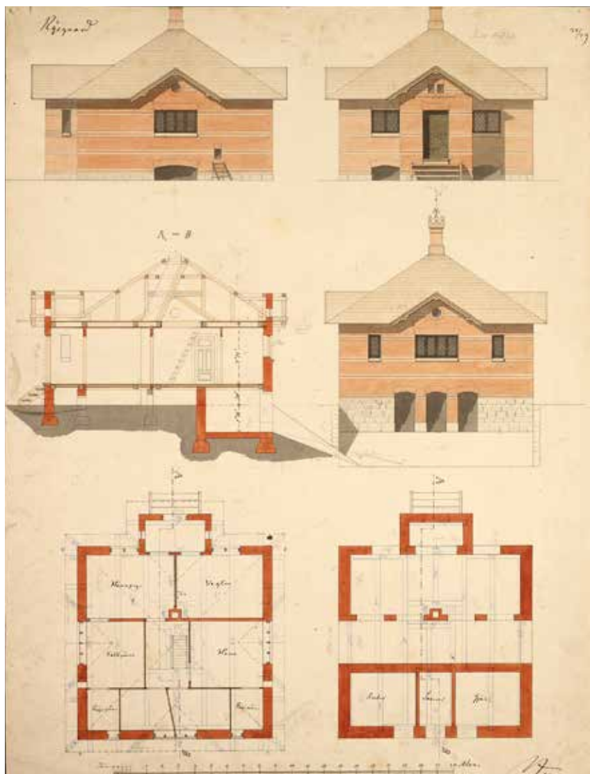
1. Frederik Vilhelm Tvede: Originaltegning til Ryegaards høsehus, 1878. Nord nedad. Det Kgl. Bibliotek – Danmarks Kunstbibliotek, Samlingen af Arkitekturtegninger (KBSA).
